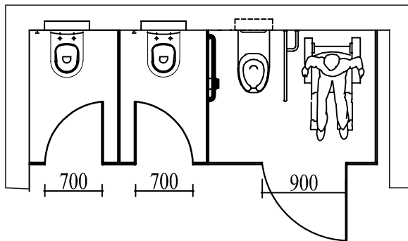
KAPI ÖLÇÜLERİ / DOOR DIMENSIONS
